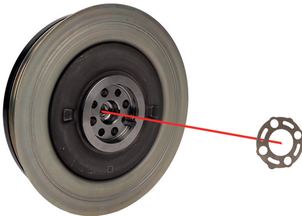
Bild 1: Kurbelwellenseite des Riemenscheibenentkopplers mit diamantbesetzter Unterlegscheibe. Bei den genannten KIT's ist diese bereits in Einbaulage am Riemenscheibenentkoppler eingelegt
