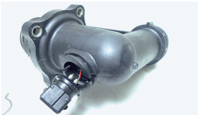
Εικόνα 2: Θερμοστάτης χαρακτηριστικού πεδίου με σπασμένη σύνδεση
