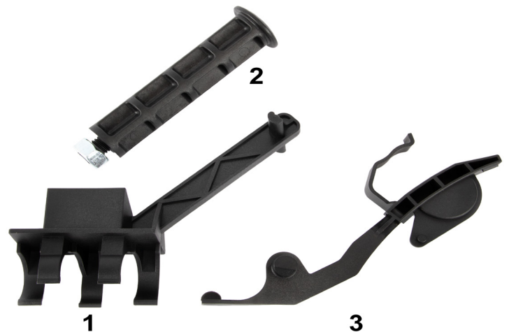
Bild 2: Montagewerkzeugsatz mit der Artikelnummer 400 0537 10
