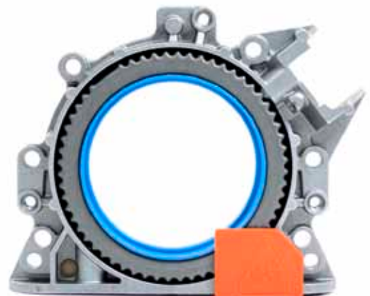
Abbildung 1_Integrierter Wellendichtring
