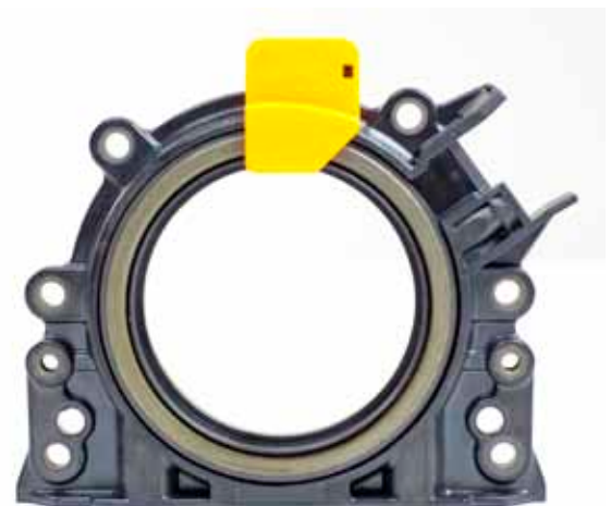
Abbildung 2_Integrierter Wellendichtring
