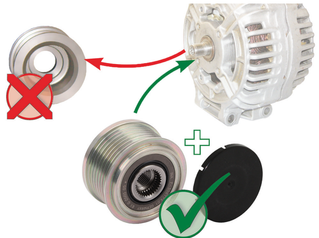
Wechsel von starrer Riemenscheibe auf einen Generatorfreilauf
