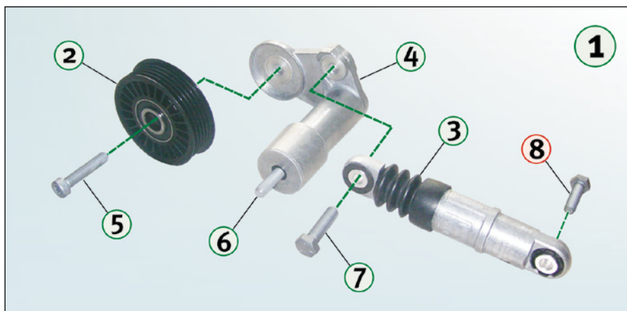
Bild 1: Detaildarstellung von 534 0014 10 mit allen Komponenten
