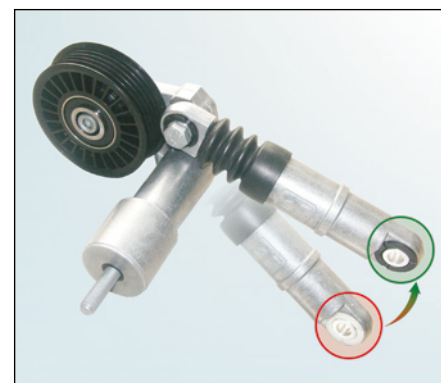
Bild 2: 534 0014 10 - Ausführung mit weißen und schwarzen Kunststoffaugen am hydr. Dämpfer
