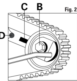
FIGURA 2 Allentare il bullone di bloccaggio B e ruotare il tendicinghia in senso antiorario; allineare l'indicatore C al centro della zona di controllo D e serrare, quindi, il bullone di bloccaggio B.
