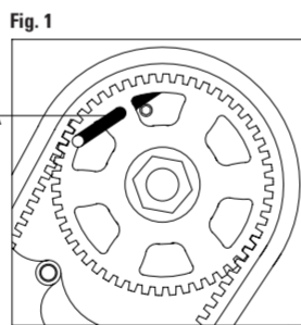
FIGURA 1 Inserire l'apposito attrezzo di bloccaggio dell'albero a camme A.
