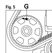
FIGURA 5 Insertar la herramienta específica para inmovilizar la polea de la bomba de inyección G.
