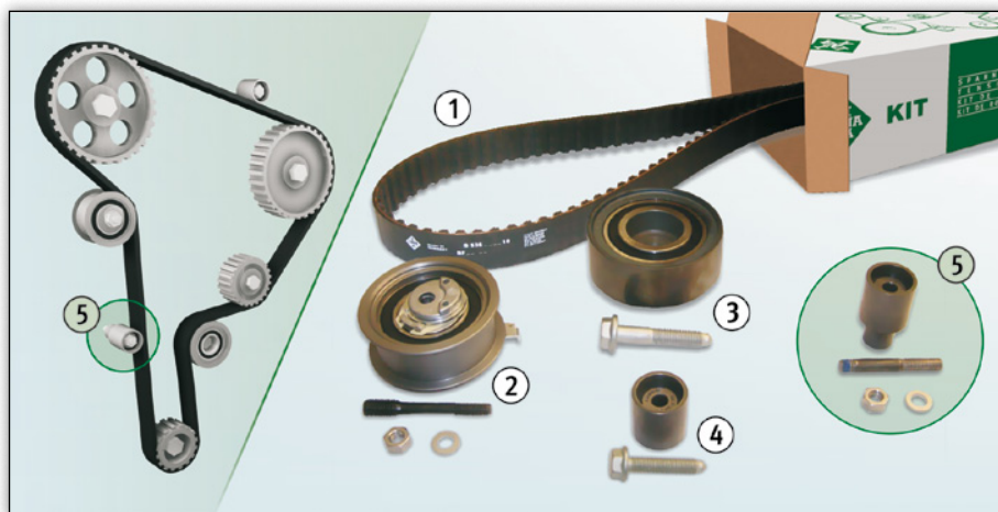
Bild 1: Triebschema 1.9 TDI/SDI und Packungsinhalt KIT 530 0361 10/530 0082 10
